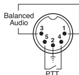
C 0376 5 Pin DIN Wiring Diagram
