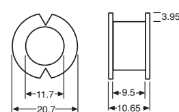
L 5305 Bobbin
