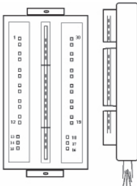
Connection stud (switchboard-riser)
