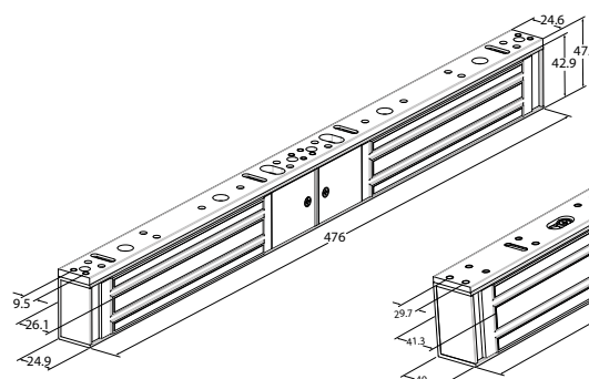
Z4 Electromagnetic Lock
