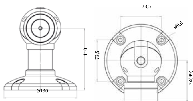
EM 830 Magnet Dimensions
